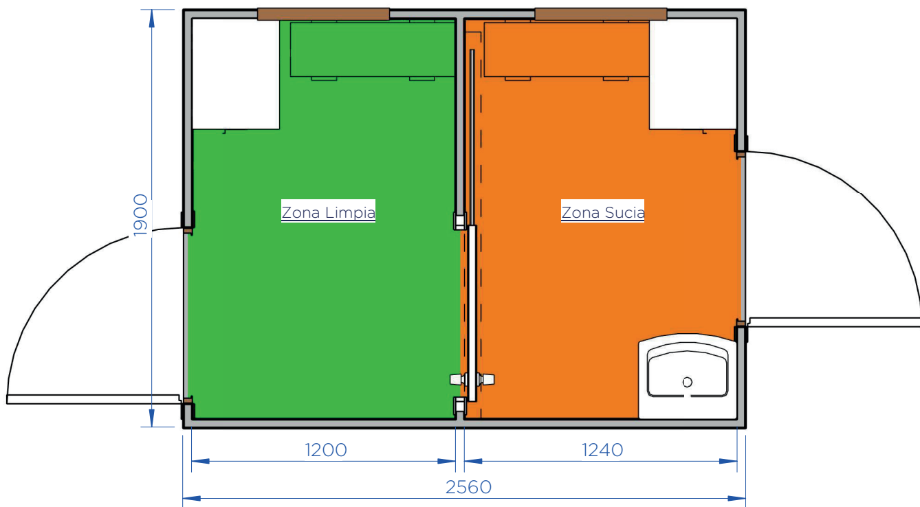
1 Planta SAS 2 2 1: 25
