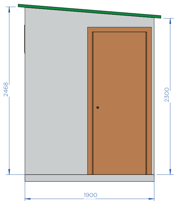
2 Alzado SAS 2 2 1: 25
